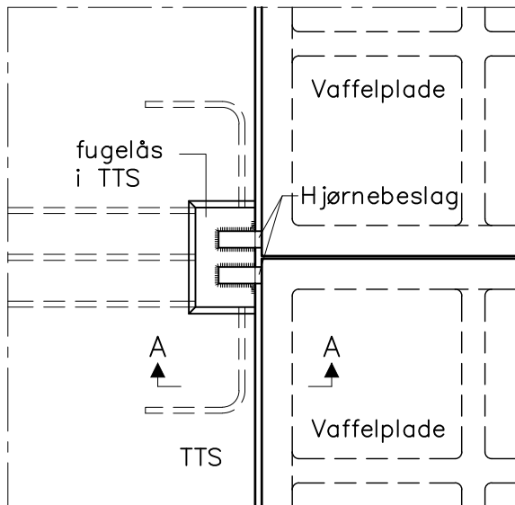
Detail 1 – hjørnebeslag
