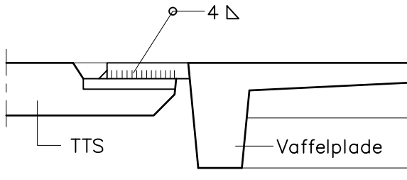
Snit A-A
