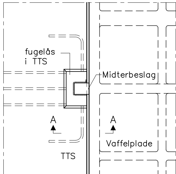
Detail 2 – midterbeslag
