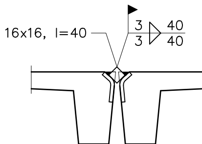
Snit B-B
