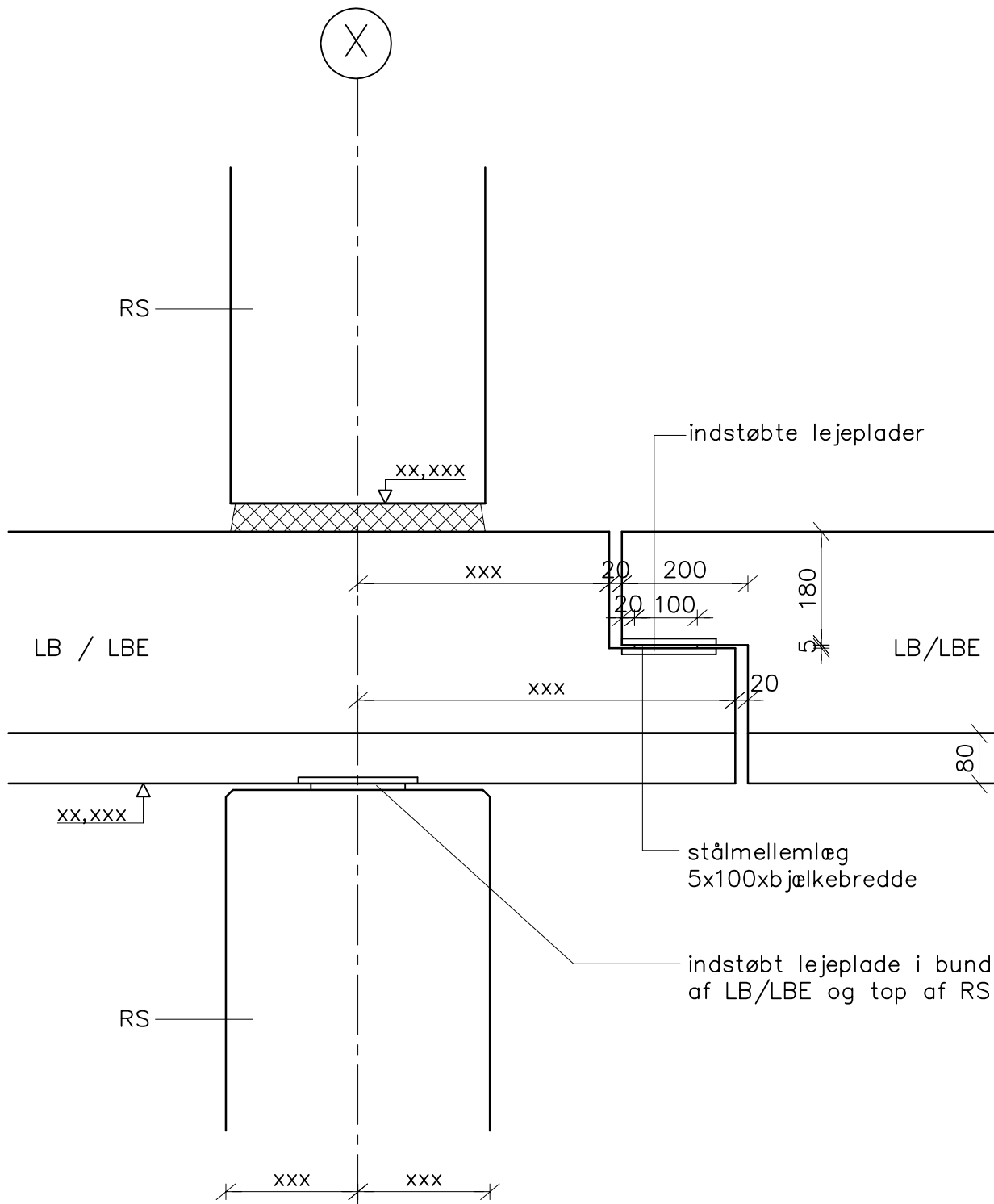
Samling mellem RS/PX/LB og LBE (etagekryds) Endesamling af LB/LBE med sadelhak.
